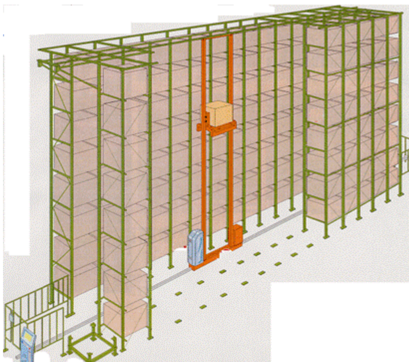
図9 自動ラック
