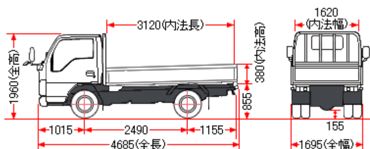
図 10 小型（2 トン）トラック（標準キャブ標準ボディ）
