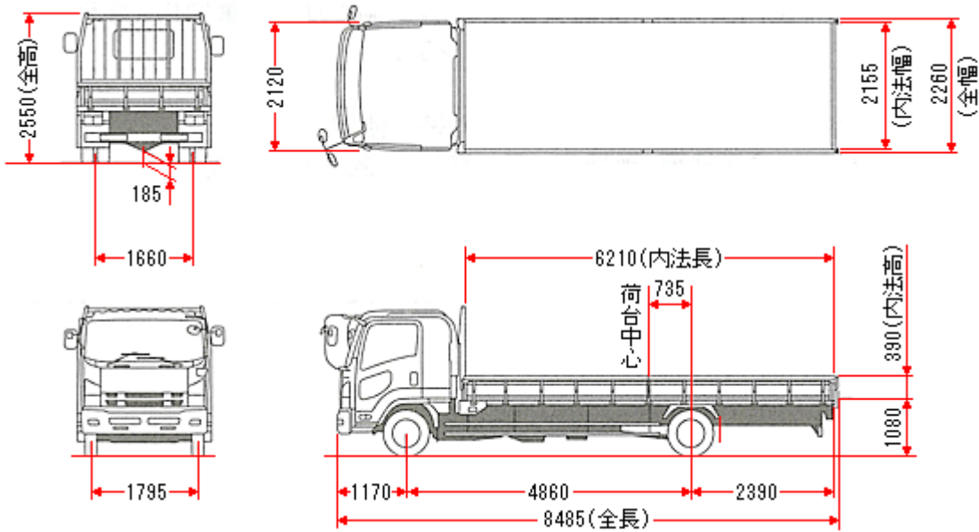
図 11 中型（4 トン）トラック（標準幅フルキャブ）
