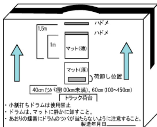
図 4 荷卸マット
