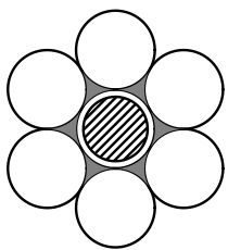
中防 ACSR/AC 25,32,58,75,80,90,95 (AL6, AC1)
